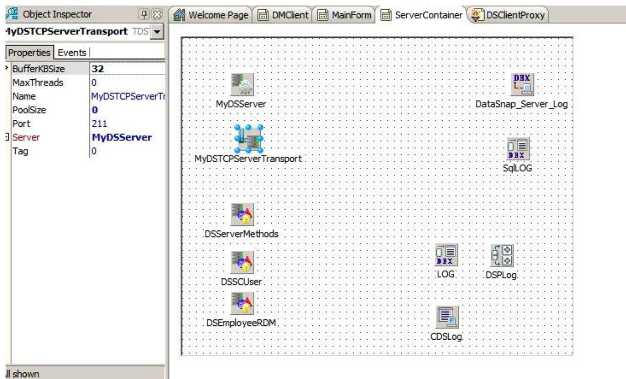
Figure 27 DSTTCPServerTransport
